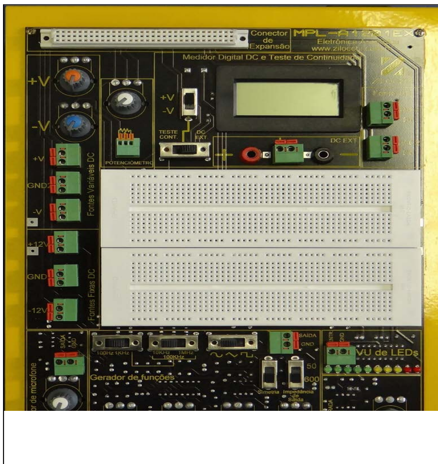
FIGURA 2 - Módulo Educacional de Treinamento para Eletrônica Analógica, modelo MPL-A1201EX, marca ZILOCCHI
